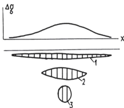
Рис. 12.4. Ілюстрація неоднозначності розв'язання оберненої задачі гравірозувідки
